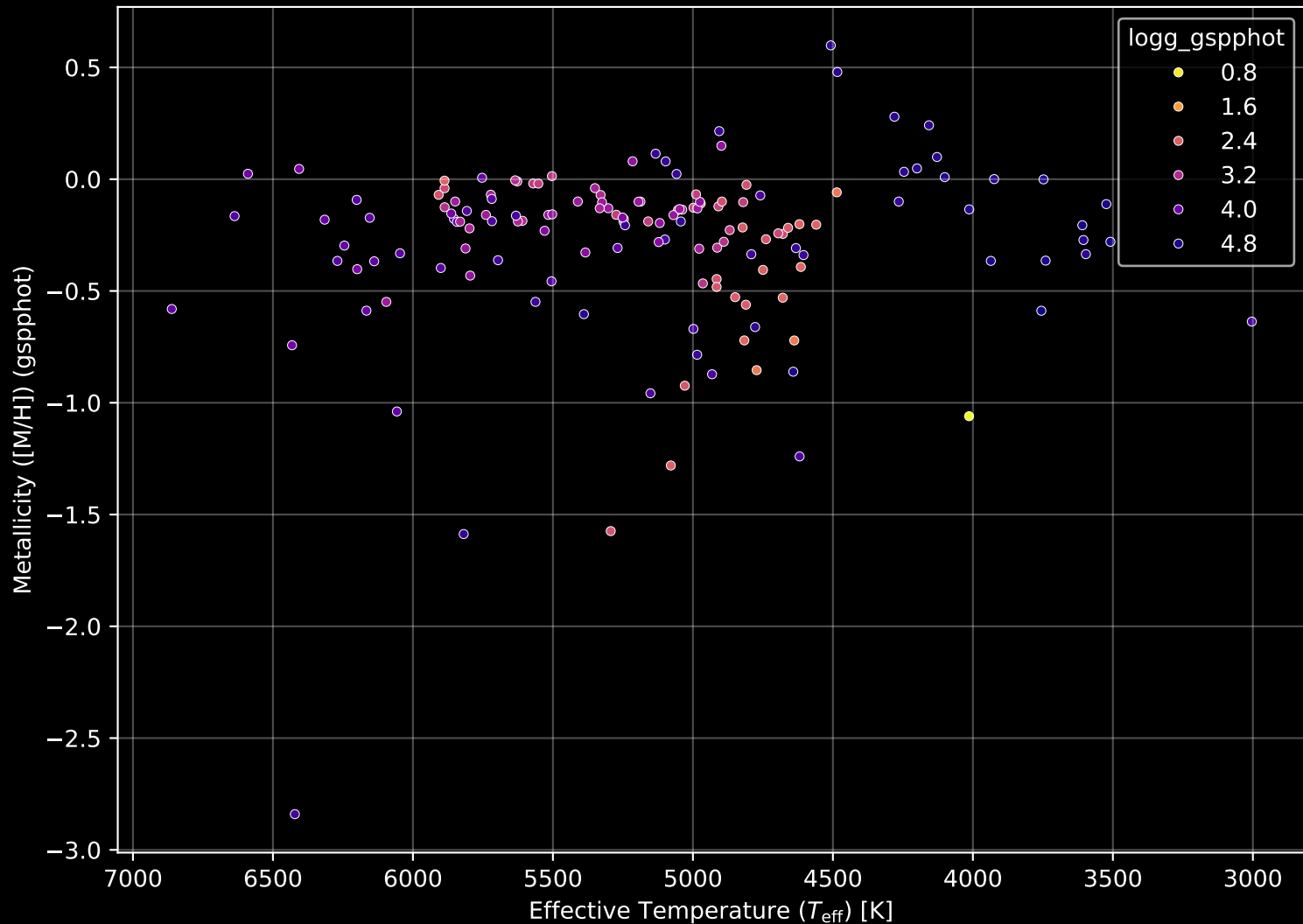
APOGEE DR17 Field: [040+60] Stellar Population Parameters (n= 150)
